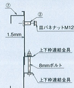
取付部詳細
